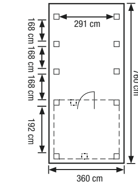
2| Mr. GARDENER Einzelcarport „Nürnberg Modern 2“ Fichte naturbelassen, mit zehn Pfosten (ca. 12 x 12 cm, 210 cm hoch) und Dacheindeckung aus Holz. Schneelast max. 125 kg pro m². (Ohne Dachpappe)
